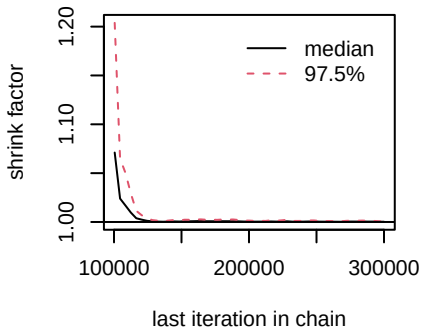
sd.d
