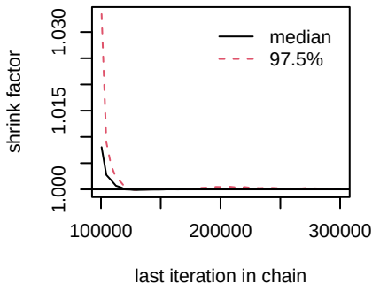
d.I.antiangio
