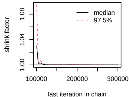
d.I.I_METi
