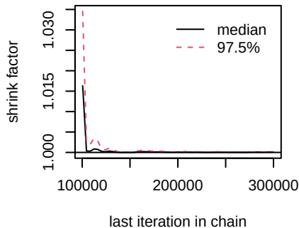
d.I.chemo
